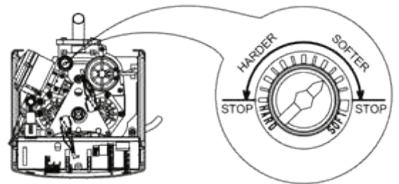
Figur 3: Sammenstikningsindstilling
